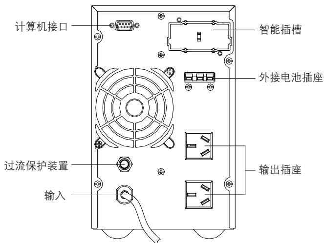
C1K(S)后盖板
