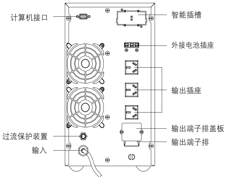
C3KS后盖板
