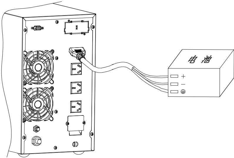
长效型UPS电池连接线示意图
