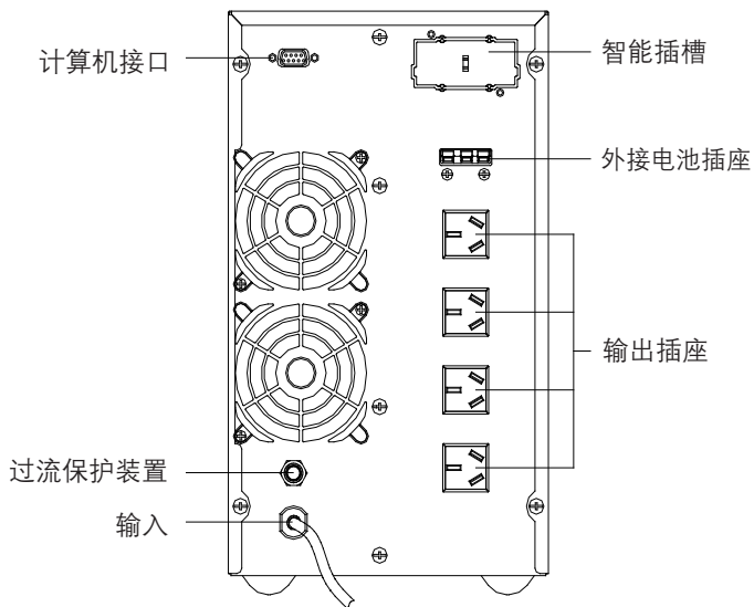
C2KS后盖板
