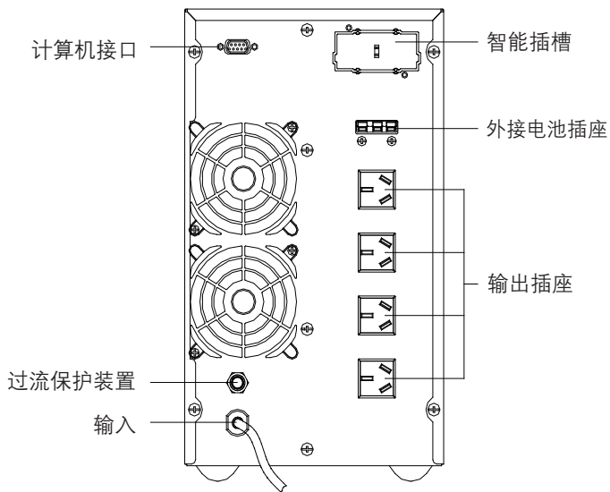
C2KS后盖板
