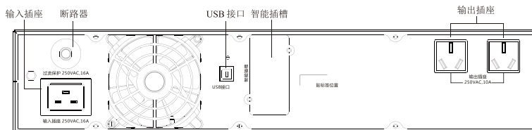
Rack2K 后盖板
