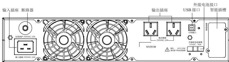
Rack2KS 后盖板
