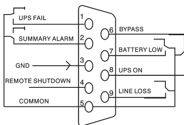
AS400 通讯界面图
