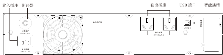
Rack1K 后盖板
