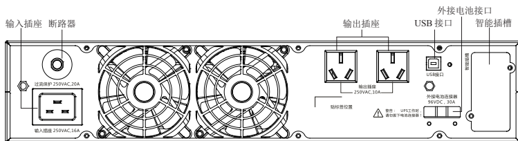
Rack3KS 后盖板
