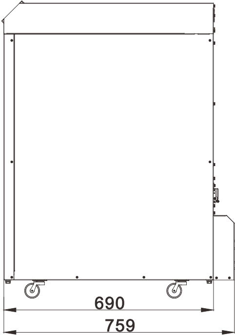
右视图
