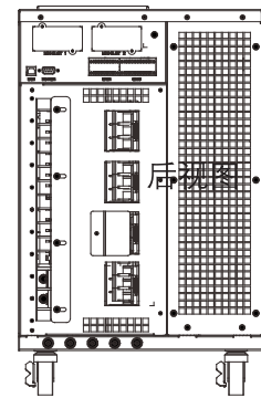
后视图
