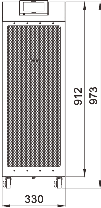
前视图
