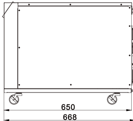
右视图
