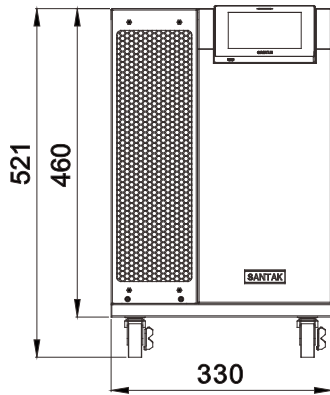
前视图
